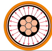
Fig. 3: Abgeschirmt mit Halbleiter Shielded cables with semiconductor
