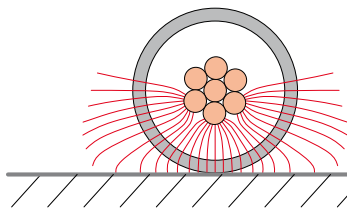
Fig. 1: Nicht abgeschirmt ohne Halbleiter Non-shielded cables without semiconductor
