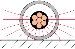
Fig. 2: Nicht abgeschirmt mit Halbleiter Non-shielded cables with semiconductor
